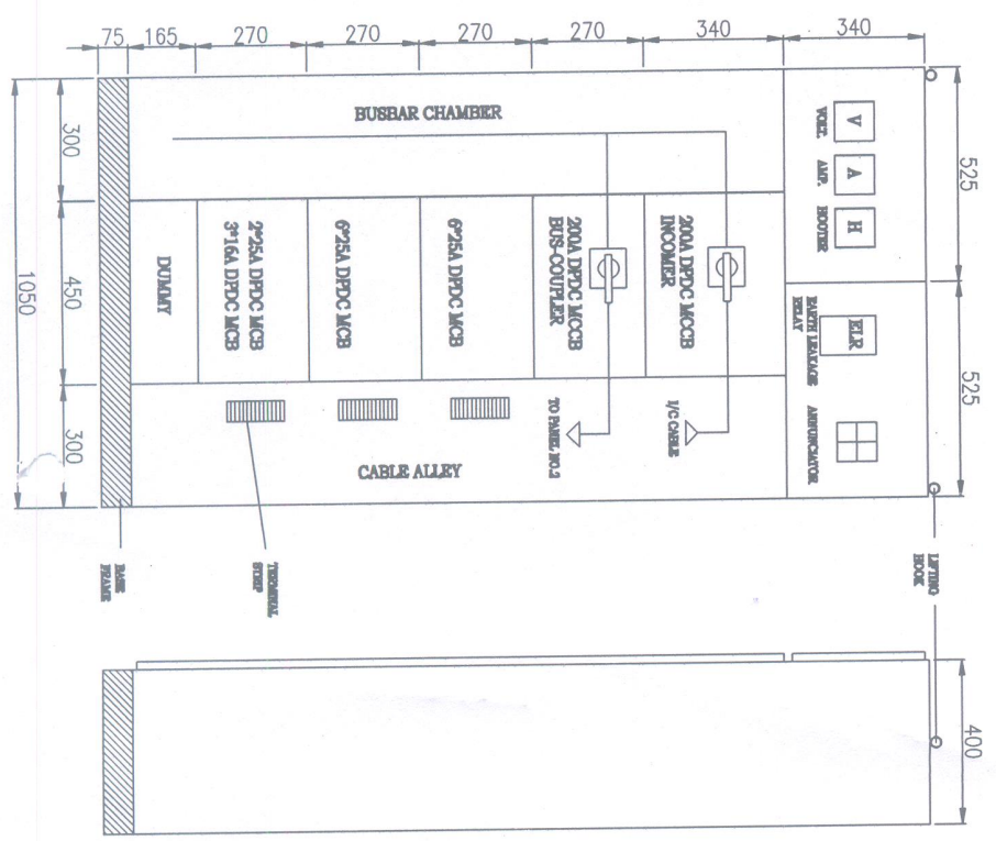
200V-200AH DCDB
